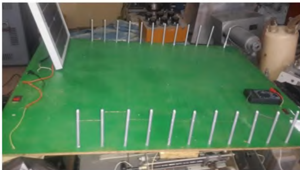
1 б – расм. Электр энергияни ўзгармас ва ўзгарувчан ток хаво линиялари орқали узатишни ўрганиш учун мўлжаланган макет.
