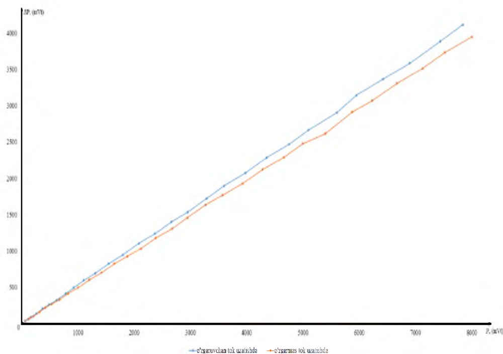
2 – расм. Ўзгармас ва ўзгарувчан токни узатишдаги қувват йўқотишларнинг узатилаётган қувватга боғлиқлиги.
