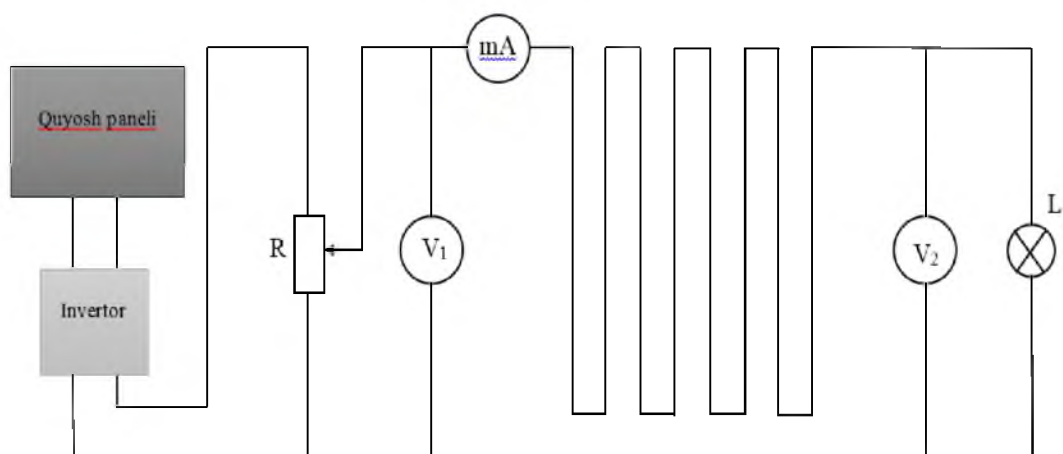
1 а– расм. Тажриба қурулмасининг схематик кўриниши.
